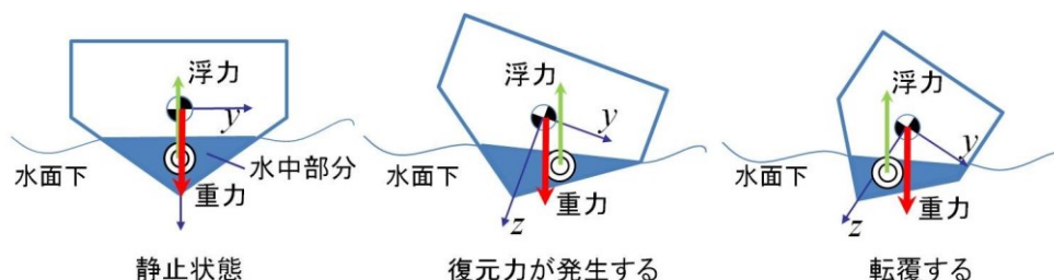
船の浮力と重力の位置関係
