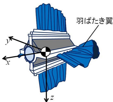
図 3-16 波動推進型生物模倣水中ロボット
