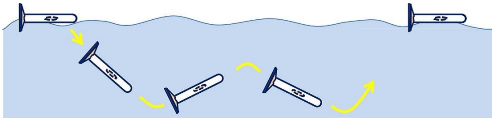
図 3-9 グライダー型水中ロボットの挙動
