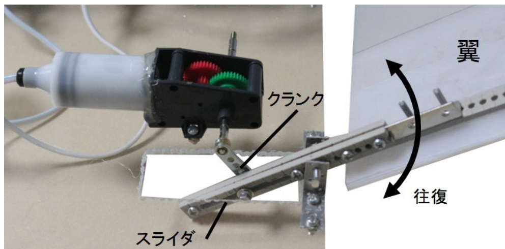
図 8-8 揺動スライダクランクによる羽ばたき機構
