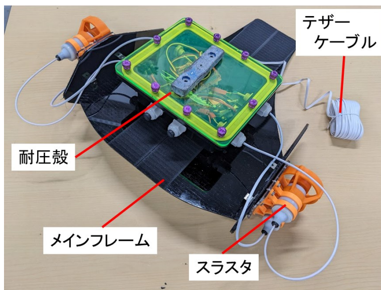
図 4-1 Mark3 概観図
