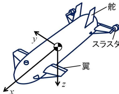
図 3-10 航行型水中ロボット
