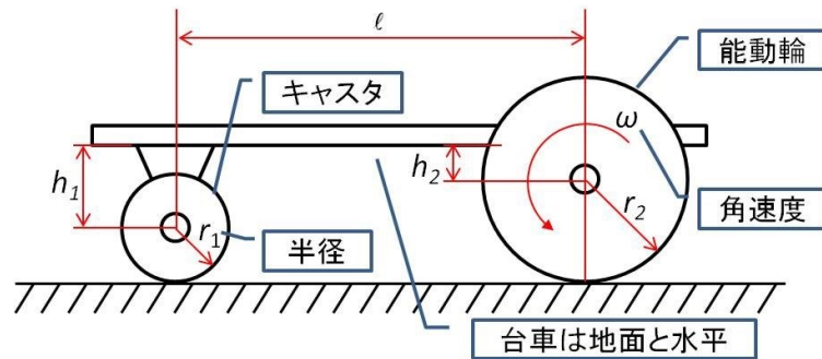
図 8-2 タイヤロボット (再掲)
