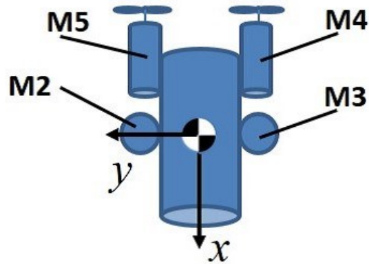
図 8-21 ホバリング型の推力配置
