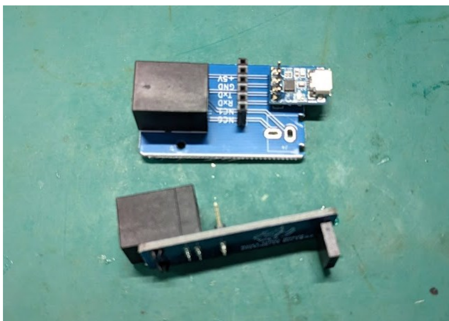
図 5-4 ジャンパを行う (JP1 と JP2 の場合)
