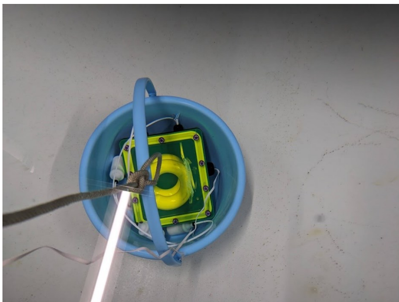
図 4-11 防水テスト
