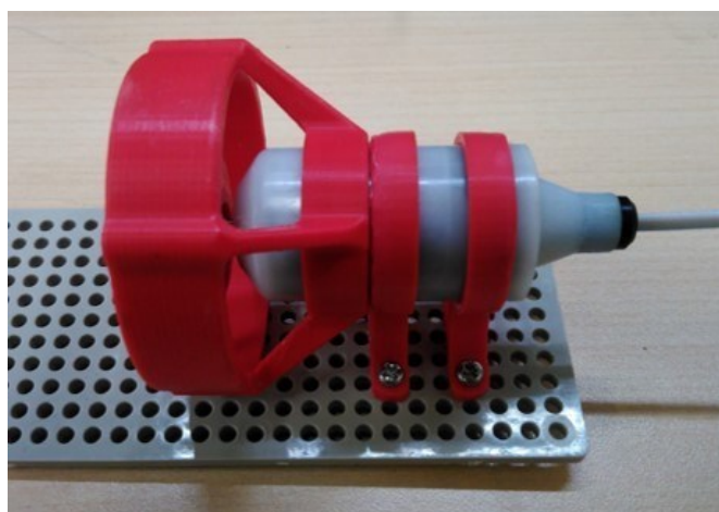
図 8-6 タミヤフレームへのスラスト固定
