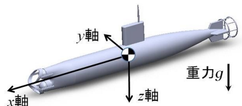
図 2-2 水中ロボットの座標系
