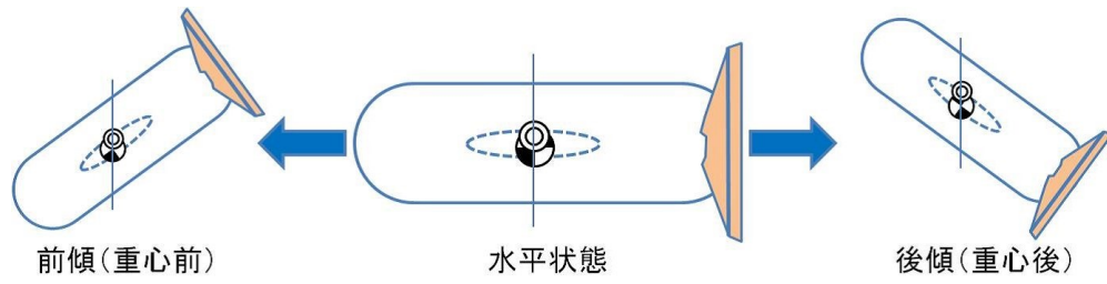
図 3-8 重心位置による姿勢変化
