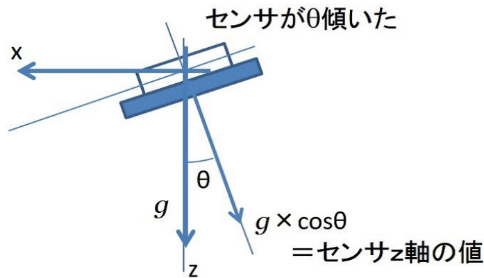
図 8-21 加速度センサで角度を取得する
