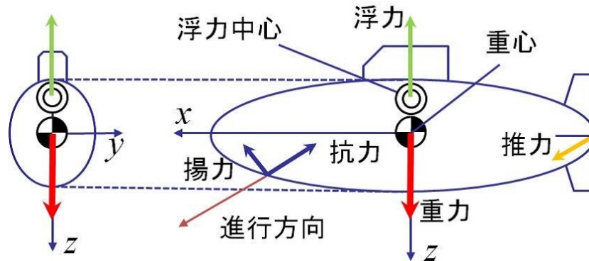
図 2-13 等速直線運動する水中ロボットに働く力
