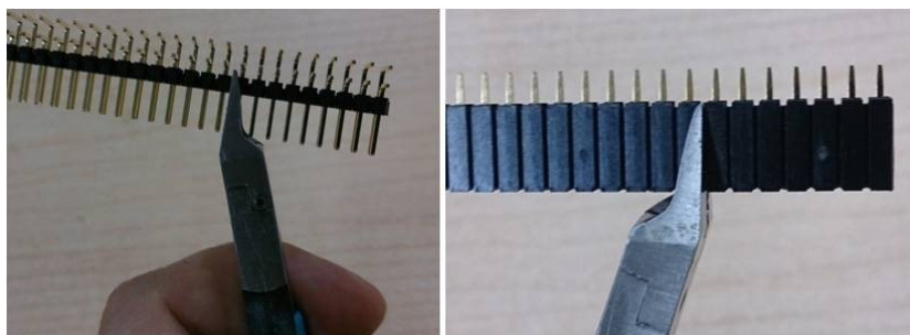
図 5-3 ピンヘッダの分割
