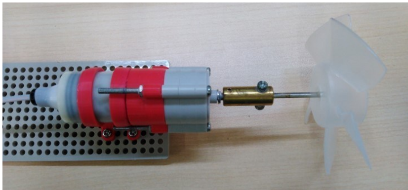
図 8-7 タミヤコネクタの使用
