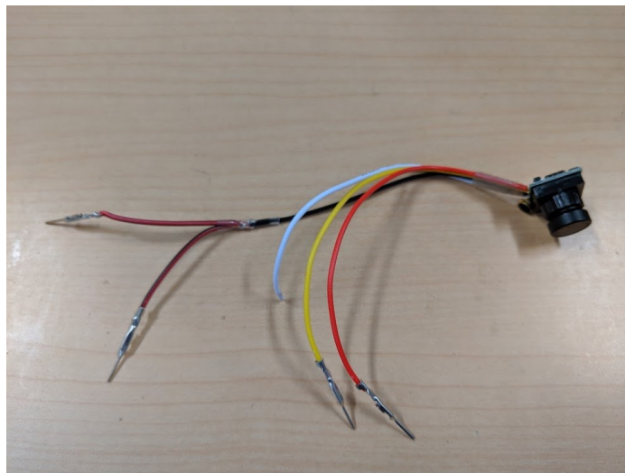
図 8-13 アナログカメラ
