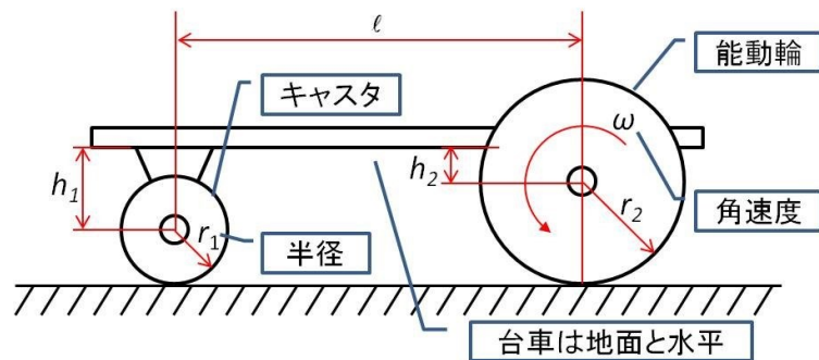
図 8-22 タイヤロボット（再掲）
