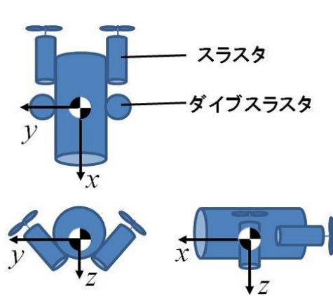
図 3-13 Z 軸移動と Y 軸移動の連成
