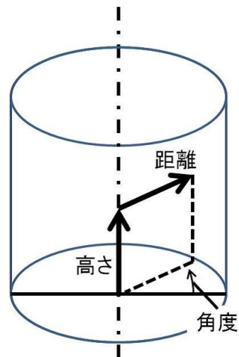
円筒座標系
