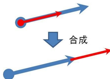
図 2-4 同軸上のベクトル合成
