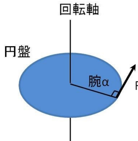
図 2-11 力のモーメント
