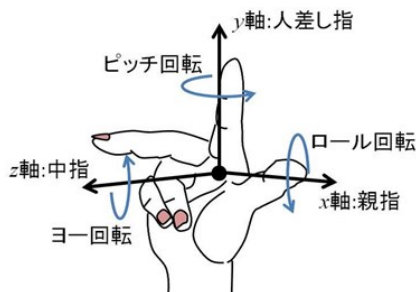
図 2-1 右手系
