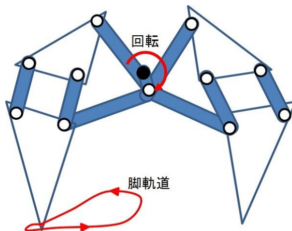
図 8-12 テオヤンセンリンク
