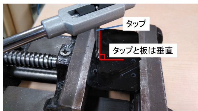
図 4-14 タップを切る
