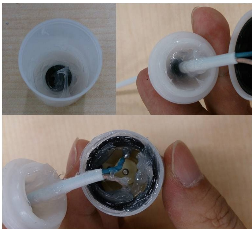
図 4-11 グリスの塗布
