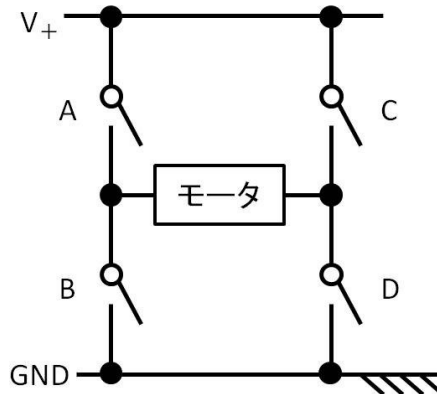
図 5-2 H ブリッジ
