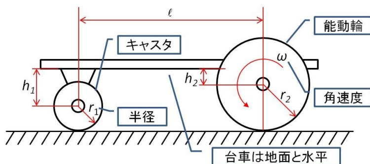
図 1-1 タイヤロボット
