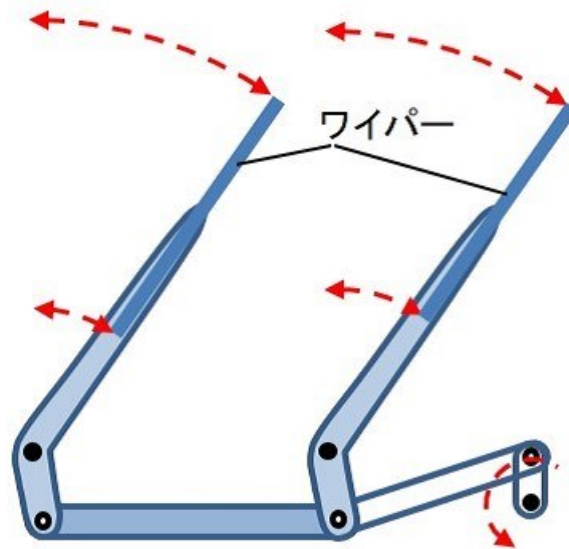
図 8-11 揺動クランク
