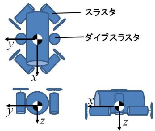
図 3-14 全方向に移動可能なスラスタ配置
