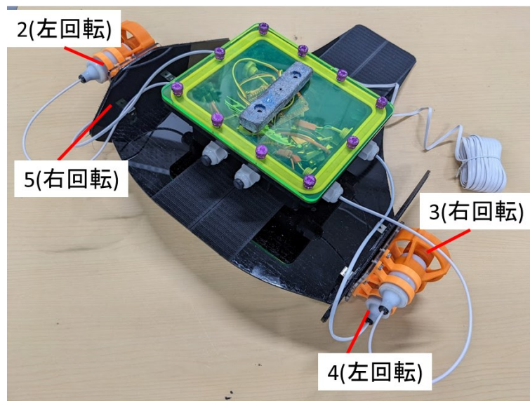
図 6-8 スラスタの配置
