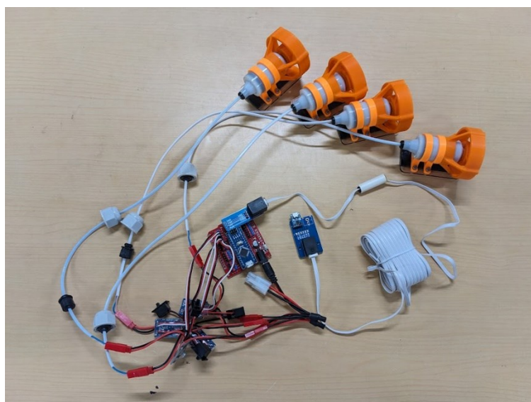
図 6-6 回路の接続
