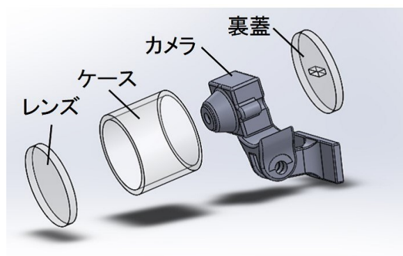
図 8-17 防水ボックスの構造
