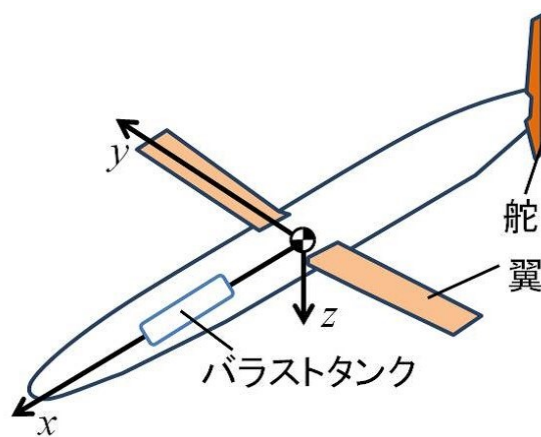
図 3-7 グライダー型水中ロボット
