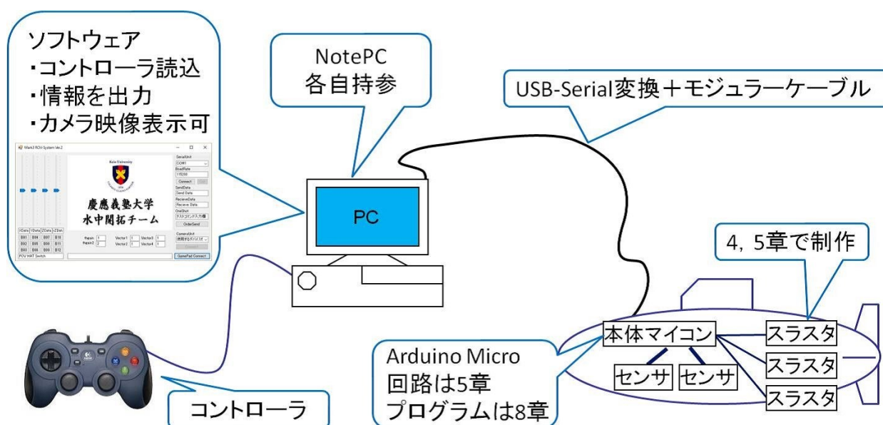
図 6-1 Mark3 と機体の接続図
