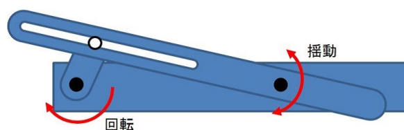
図 8-9 揺動スライダクランク
