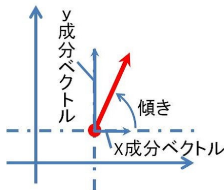
図 2-5 ベクトルの分解
