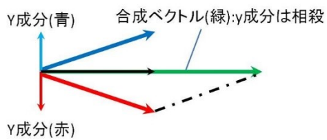
図 2-7 ベクトルの合成 2
