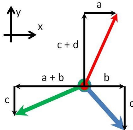
図 2-10 3つのベクトルの合成
