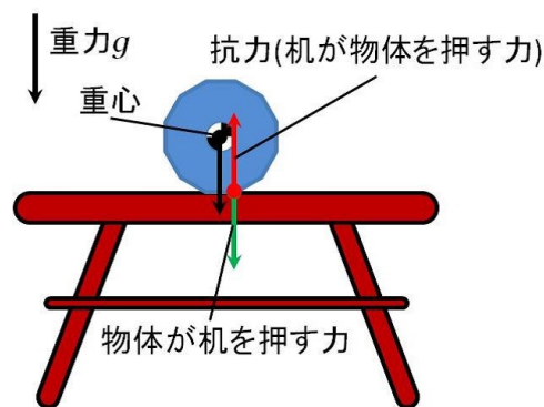
図 2-9 机と物体の作用反作用
