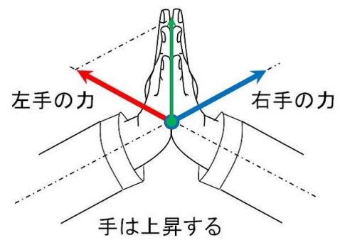
図 2-8 ベクトル表記
