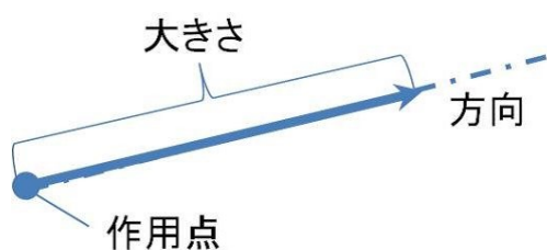
図 2-3 ベクトル表記
