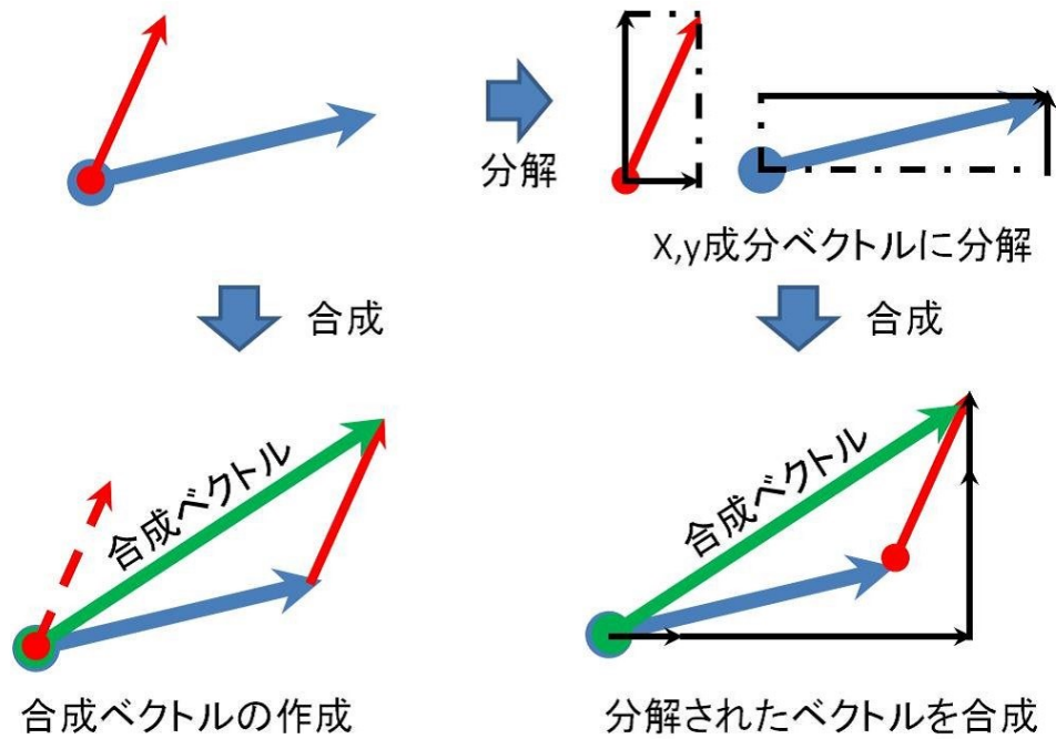
図 2-6 ベクトルの合成と分解
