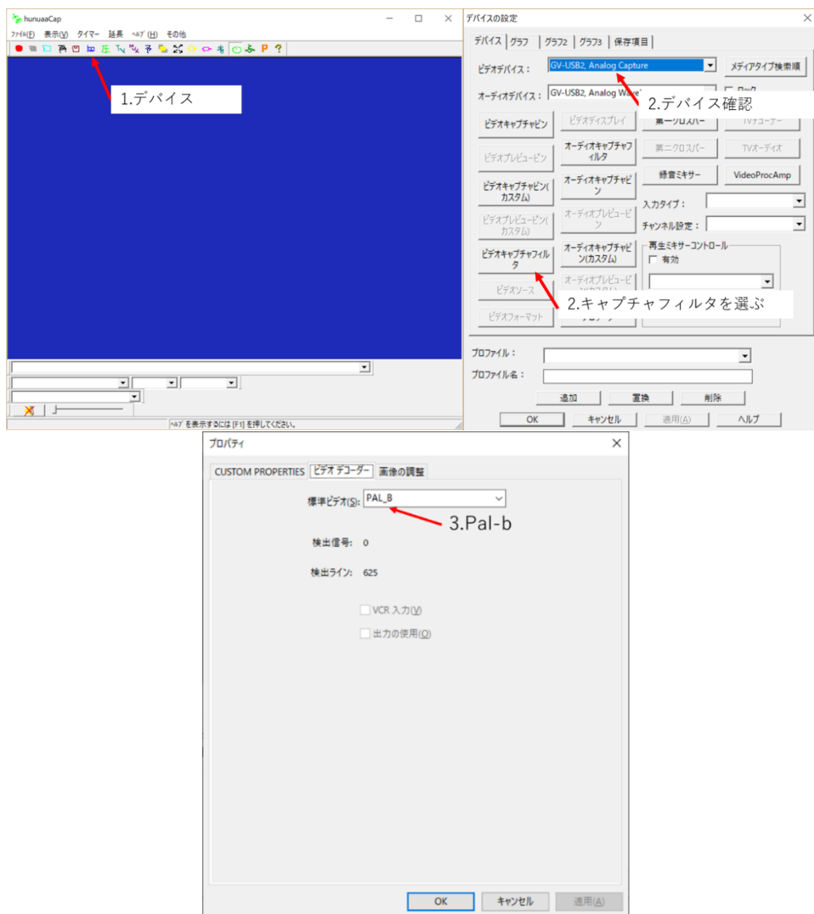
図 8-15 hunuuaaCAP の設定
